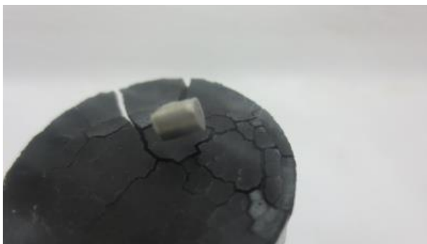
液体窒素実験（超伝導現象の観察）
